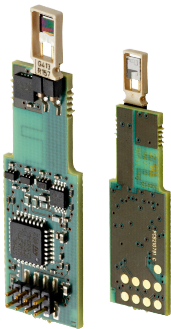
HTM10SP 相对湿度和温度模块
