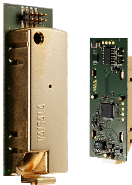
GM10SP CO 2 模块
