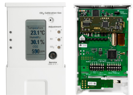
GMW95R CO 2 、相对湿度及温度变送器
