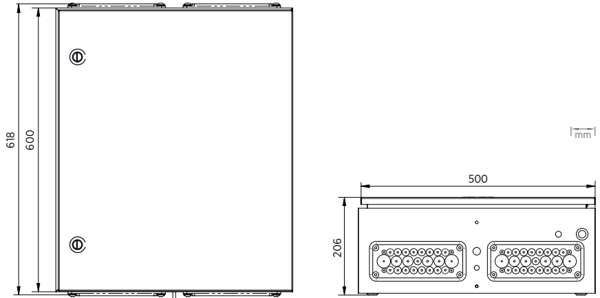
Figure 21 Dimensions du boîtier CAB100B
