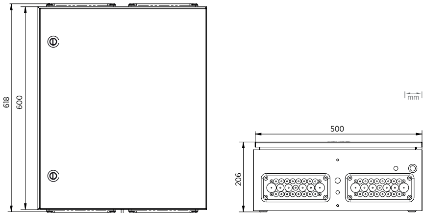
Abbildung 14 CAB100B Gehäuseabmessungen
