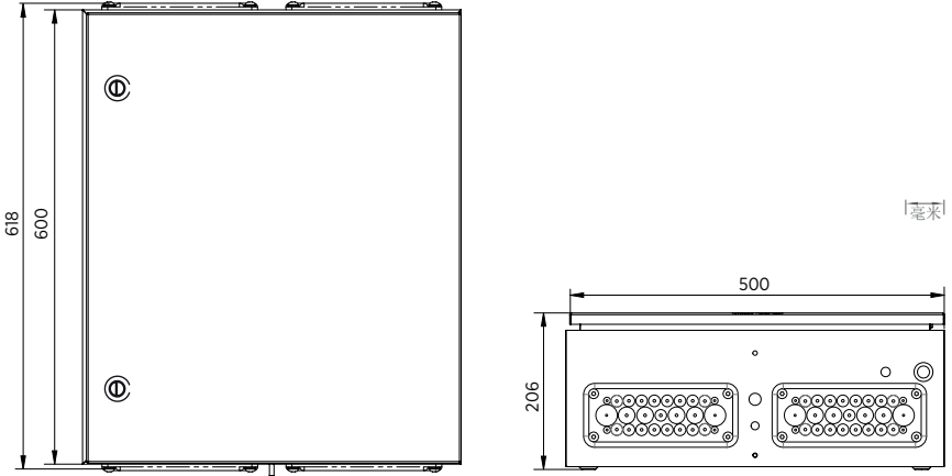
图 49 CAB100B 外壳尺寸
