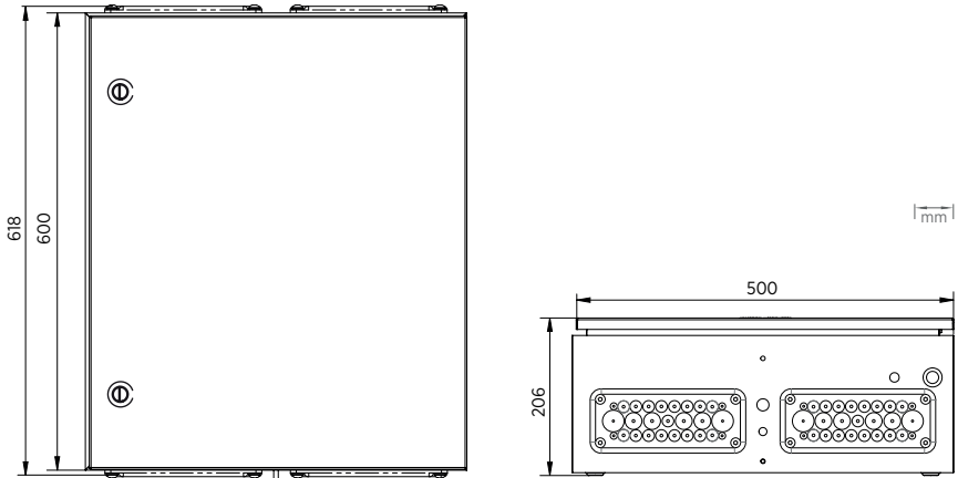
Figura 35 Dimensões do invólucro CAB100B
