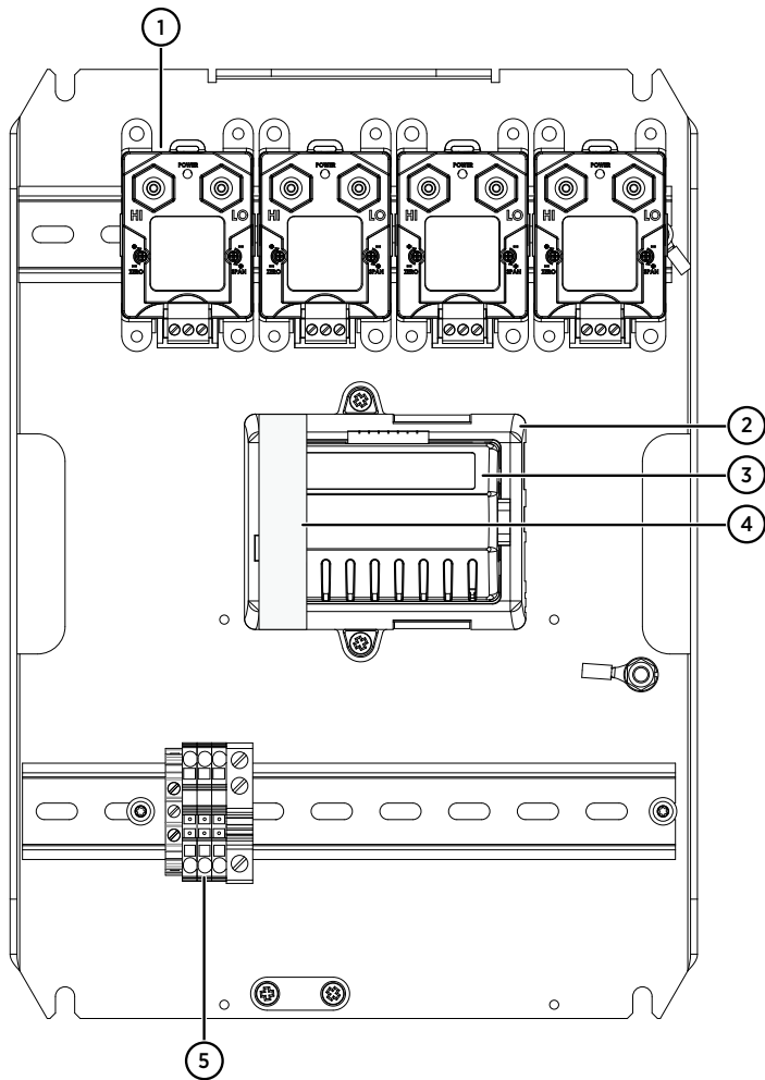
Figura 25 Componentes principales del CAB100A, modelo PDT101 con vNet PoE
