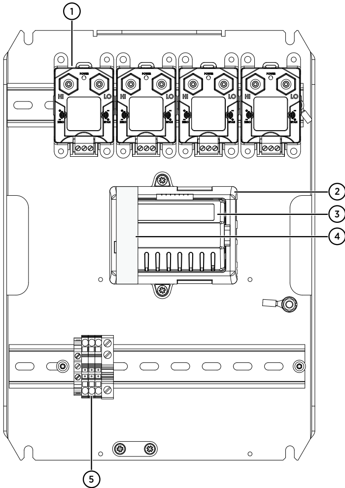
Abbildung 11 Hauptkomponenten im CAB100A, Modell PDT101 mit vNet PoE
