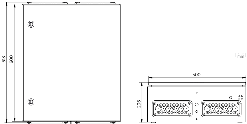
Figura 28 Dimensiones del compartimento del CAB100B
