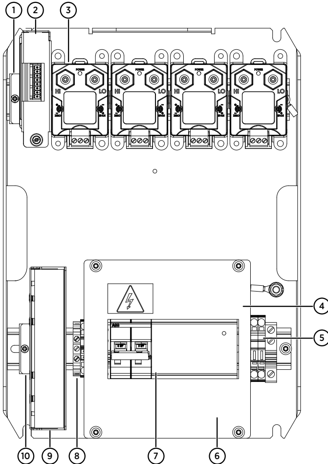
Figura 24 Componentes principales del CAB100A, modelo PDT101 con servidor de puerto serial y sistema de alimentación de 24 VCC
