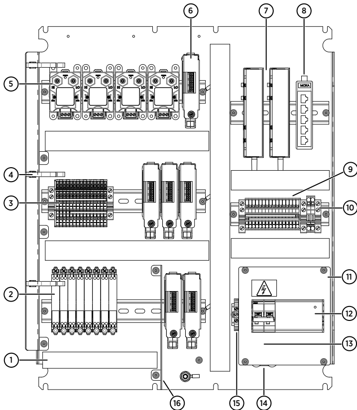
Figura 26 Componentes principales del CAB100B, modelo mixto con PDT101, canales de entrada analógica y barreras de seguridad
