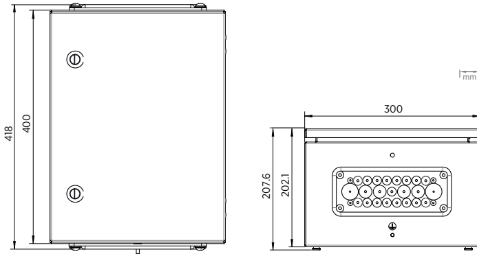
Figura 27 Dimensiones del compartimento del CAB100A
