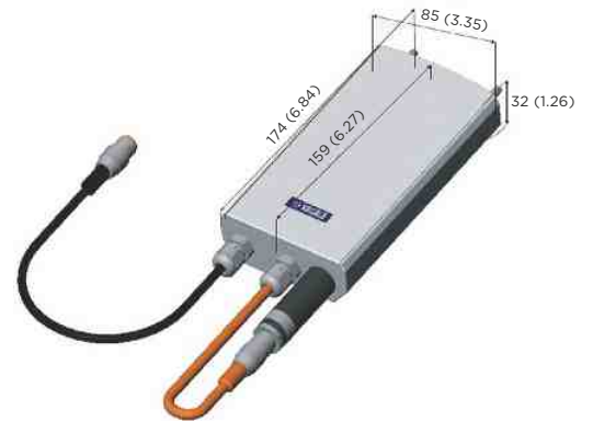
GM70 Membranpumpe mit Sonde
