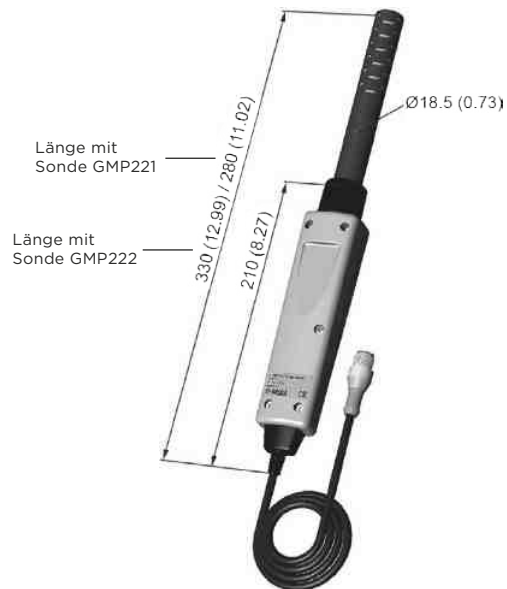
Sondengriff mit Sonde
