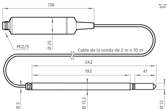
Dimensiones del DMP5
