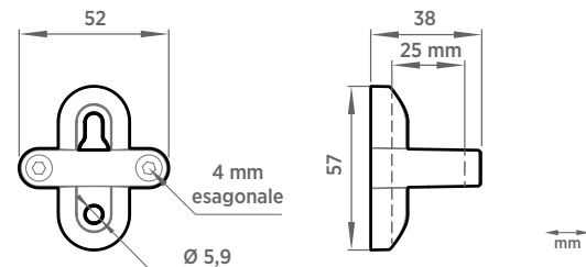
Dimensioni supporto per sonda ASM213582
