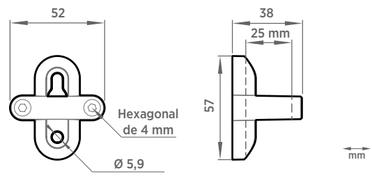
Dimensiones del sujetador de la sonda ASM213582
