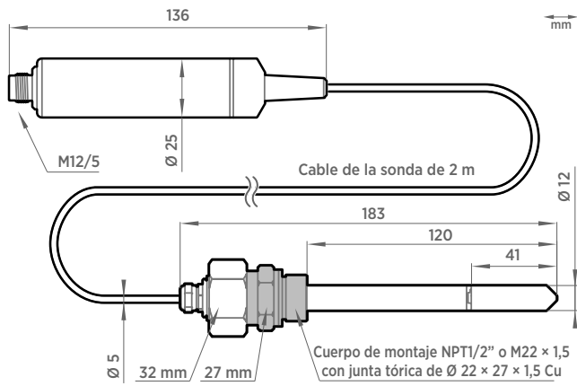
Dimensiones de la sonda HMP4
