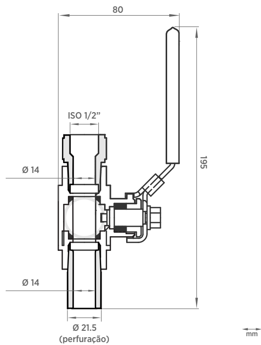
Dimensões do kit de válvula esférica
