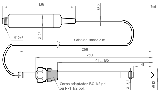
Dimensões da sonda HMP8
