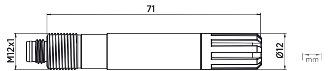
Abmessungen Kabelsonde
