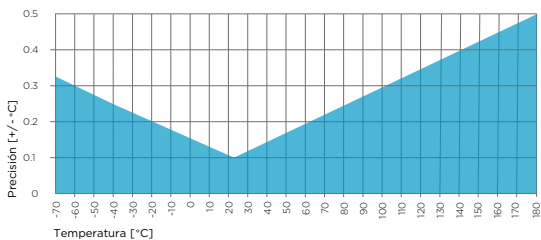
Precisión en la medición de temperatura sobre el rango completo
