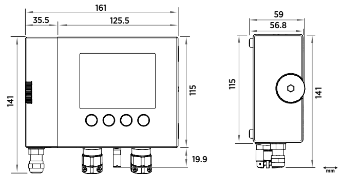
Dimensiones del HMT370EX en milímetros
