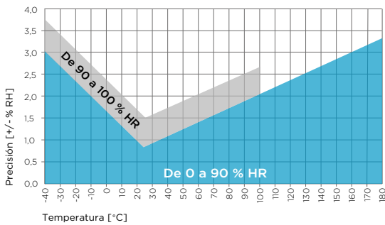
Precisión en la medición de humedad en función de la temperatura
