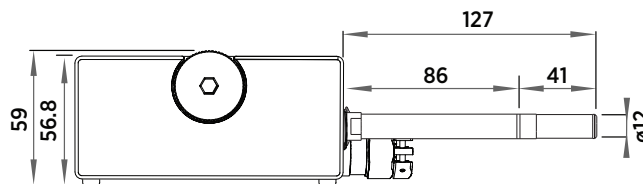
Dimensiones en mm
