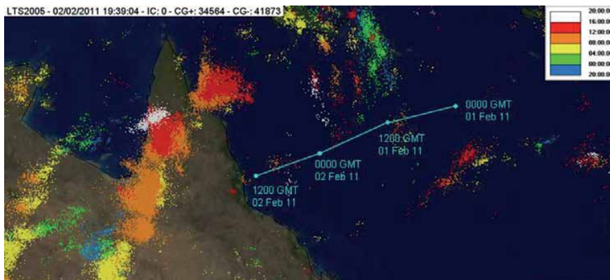
Figura 1. La trayectoria del ciclón tropical Yasi se muestra en azul claro mientras se desplaza del E-NE al O-SO, con las localizaciones señaladas a las 00:00 y 12:00 UTC del 1 y el 2 de febrero.
