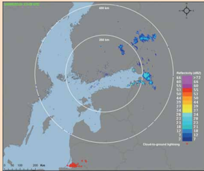
Figura 9. Reflectividad medida por el radar meteorológico WRM200 de Vaisala combinada con impactos de rayos agrupados en periodos de 15 minutos medidos por el servicio global de datos de rayos Dataset GLD360 de Vaisala. La primera detección de la tormenta (mostrada en el pie de la imagen) aproximándose a Escandinavia fue proporcionada por el GLD360.
