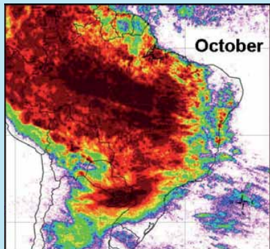
Figura 3. La cantidad de impactos del GLD360 se incrementó de 1,1 millones en junio a 3,4 millones en agosto, antes de incrementarse diez veces hasta 32,0 millones en octubre a la llegada del verano.
