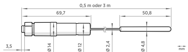
Abmessungen TMP115
