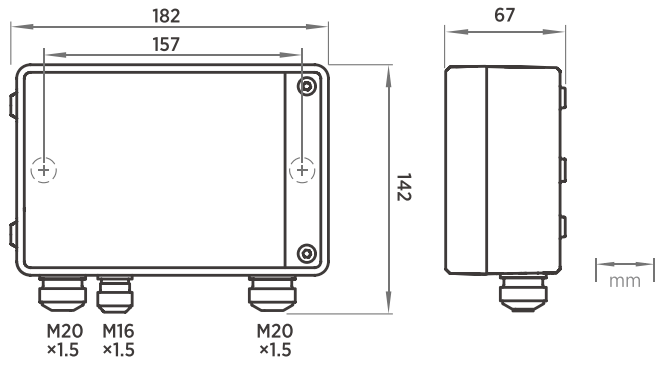
Indigo510 尺寸和接线口尺寸
