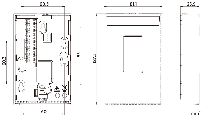
GMW83D 和 GMW83DRP 尺寸
